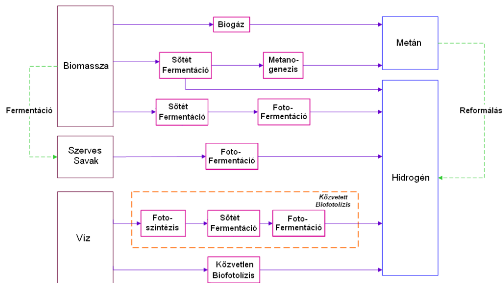
1. ábra A hidrogén előállításának lehetőségei biológiai rendszerekkel
